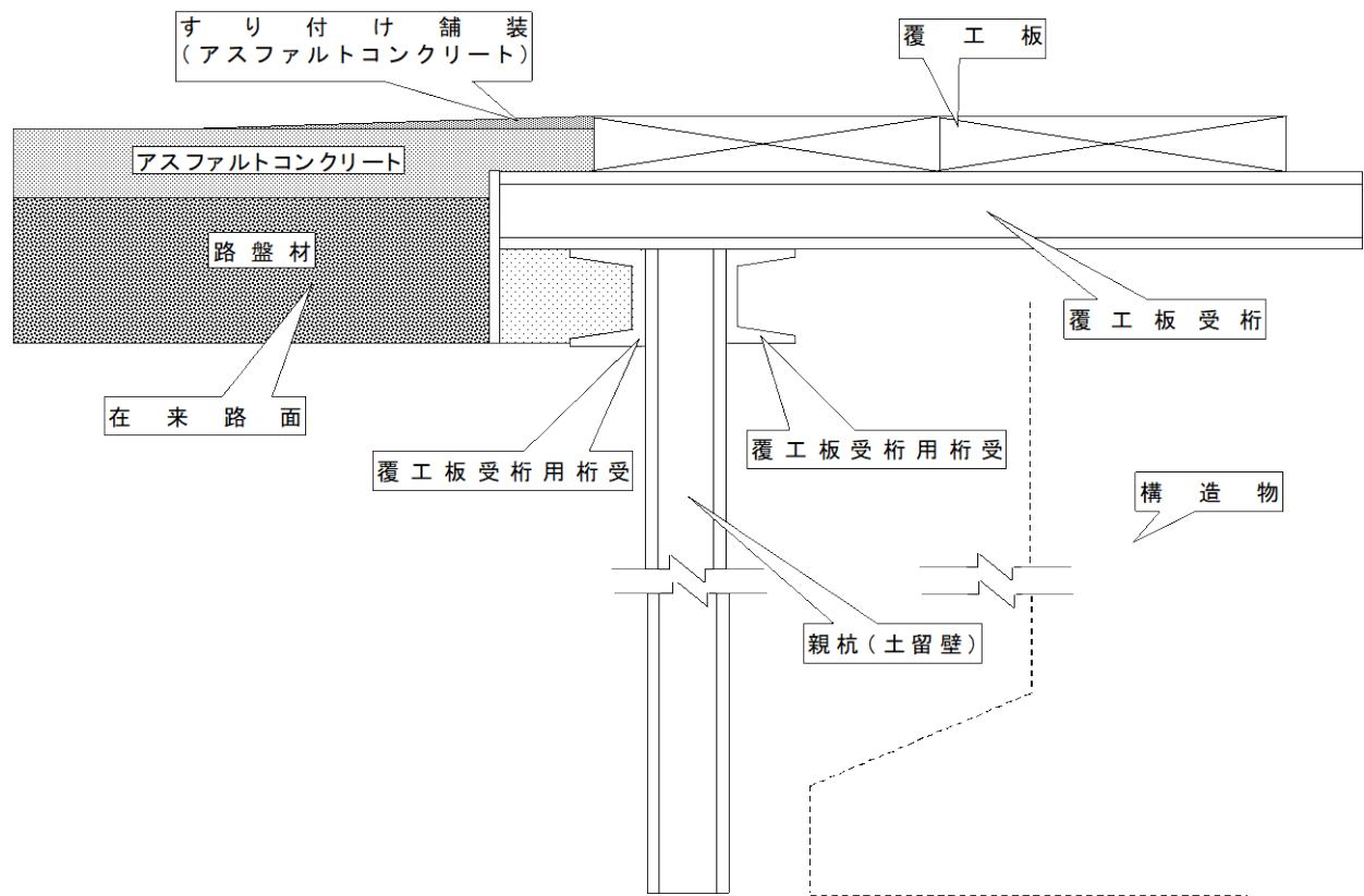
参考図（覆工板受桁および桁受）
