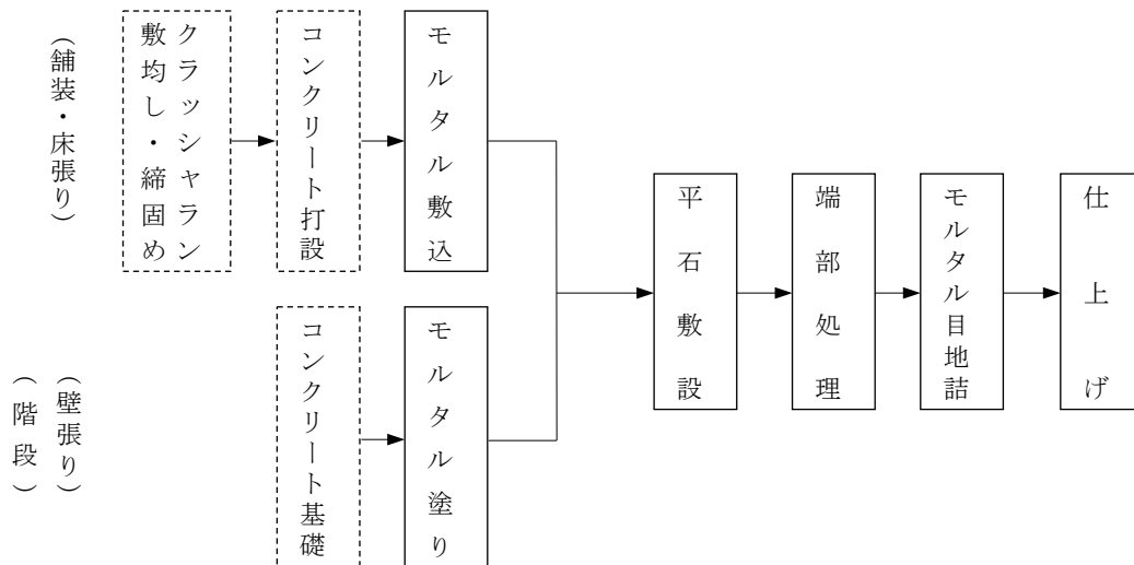
図2.1 施工フロー
