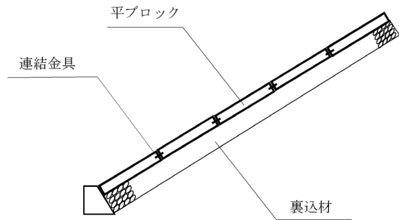
断面図
