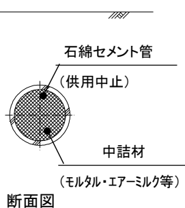
図 1 3 管路の移設
