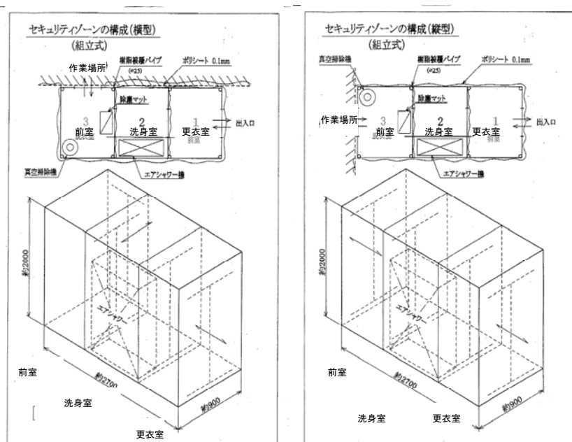
図1 セキュリティゾーンの事例
