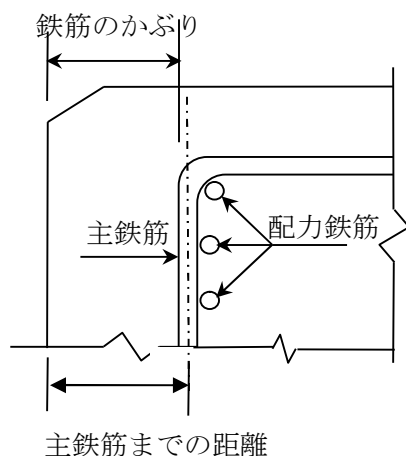
図 3-9-1 鉄筋のかぶり
