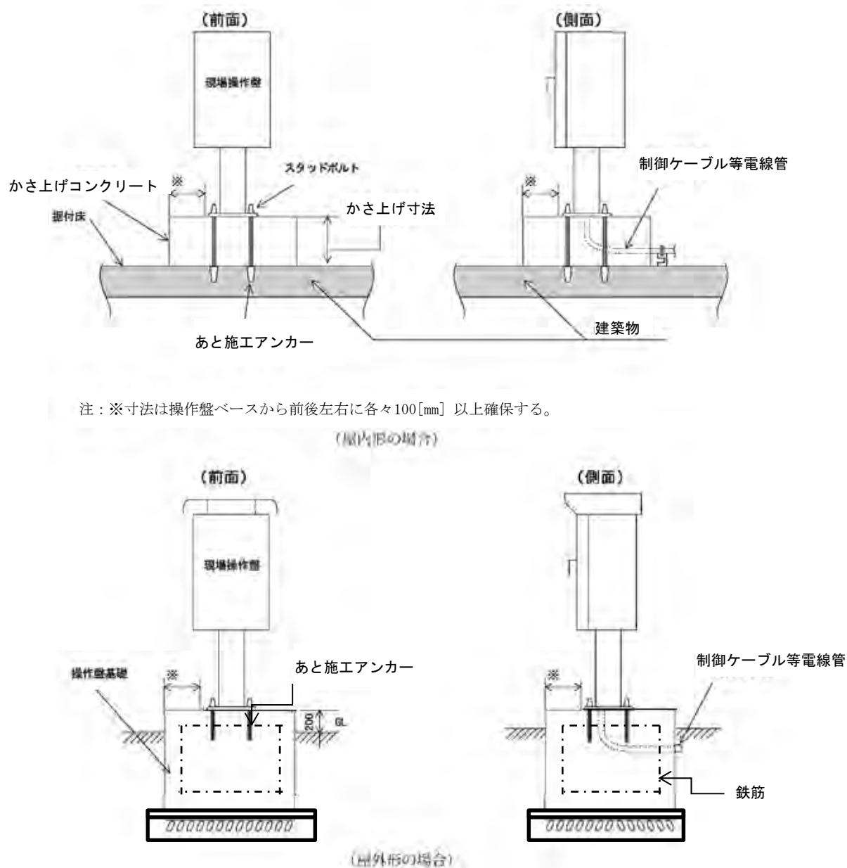
図 4.2-4 現場操作盤施工例
