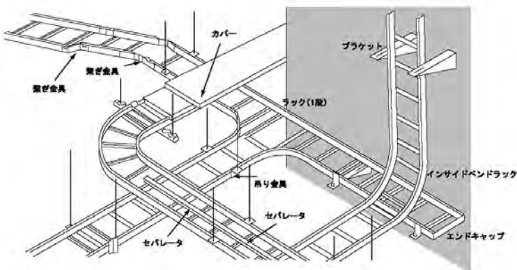
図 4.1-7 ケーブルラック工事（例）
