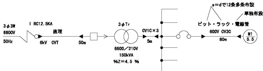
図 4.3-6 選定回路例
