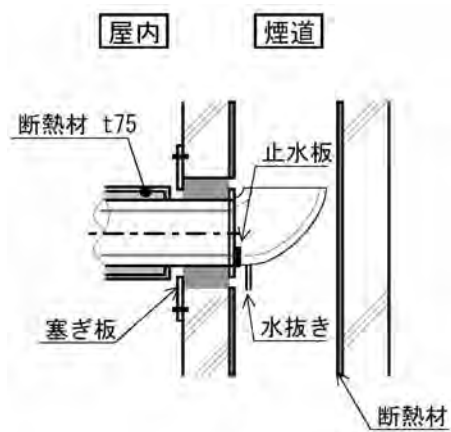
図 4.2-9 煙道への接続法
