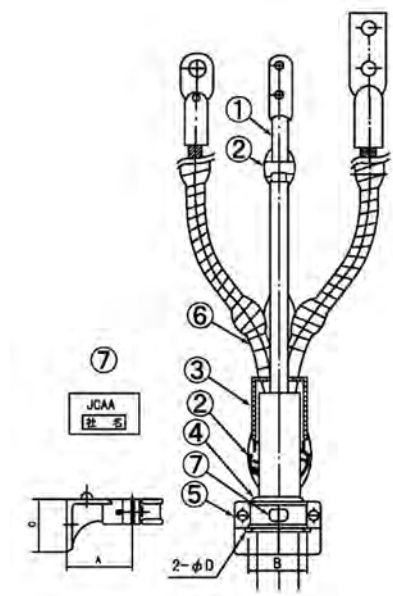
図 4.3-2 テープ巻形屋外終端処理図「参考図」 (600 V 3心 CV用) (JCAA規格 C4102 (屋内)、C4103 (屋外))
