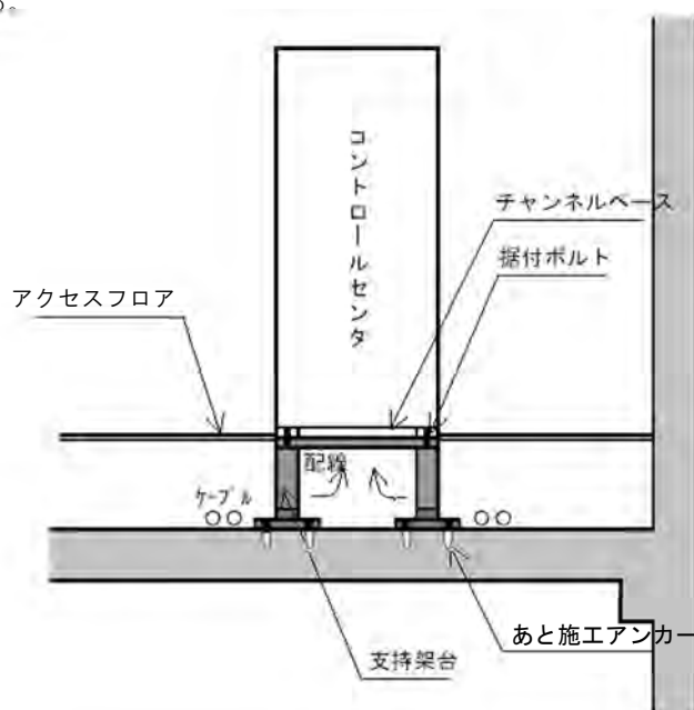
図 4.2-3 コントロールセンタ施工図例
