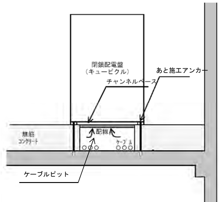
図 4. 2-1 閉鎖配電盤施工図例
