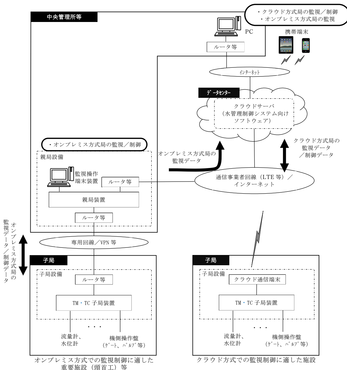
図 1.2-2 ハイブリッド方式の水管理制御システムの概念図
