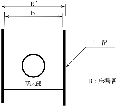
図2-4 土留施工の床掘幅（砂・砕石基礎）
