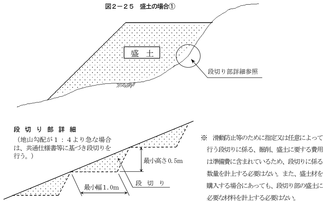
図2-25 盛土の場合①
