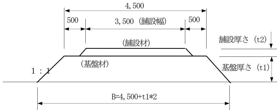
図15-17 標準断面図
