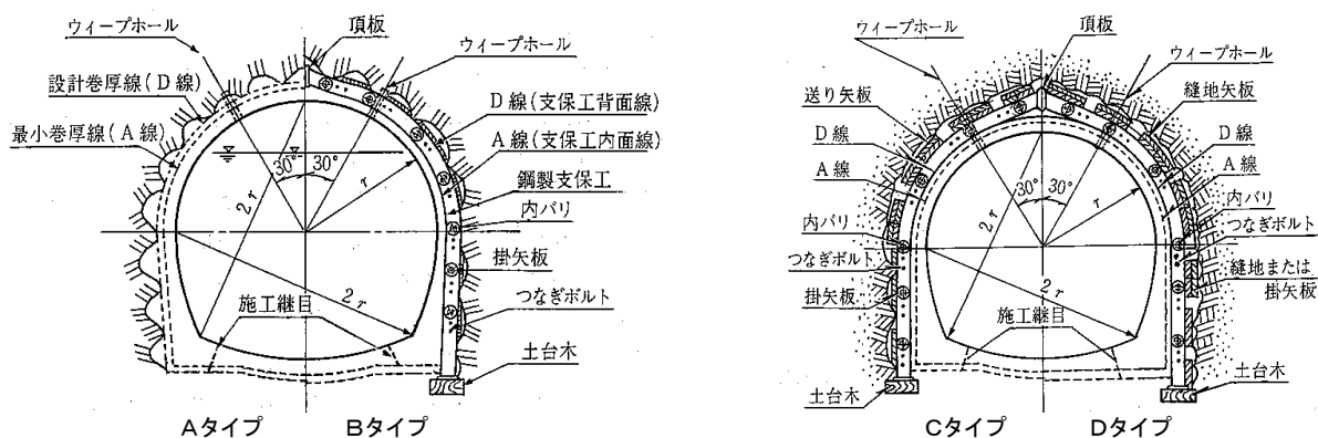
矢板工法標準断面図（標準馬てい形の場合）
