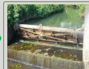
施工前
