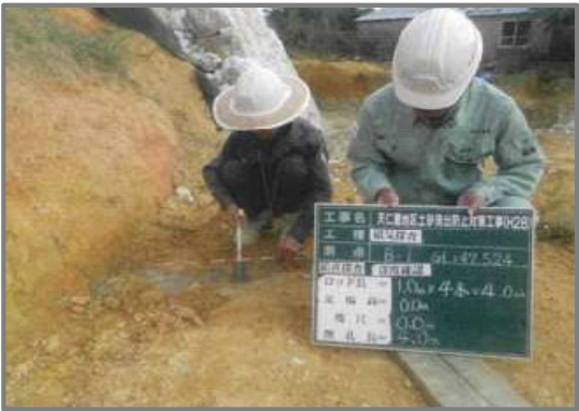
鉛直探査
