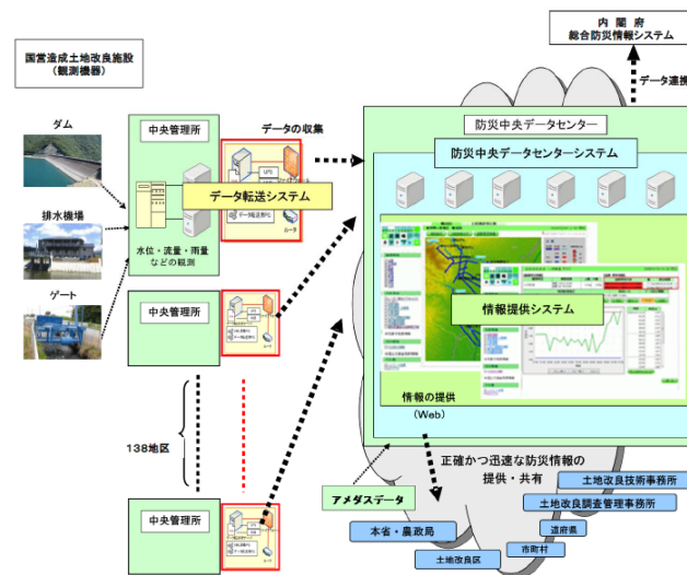
【国営造成土地改良施設防災情報ネットワークの概念図】
