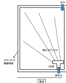
集水溝+弾丸暗渠+額縁明渠の施工図
