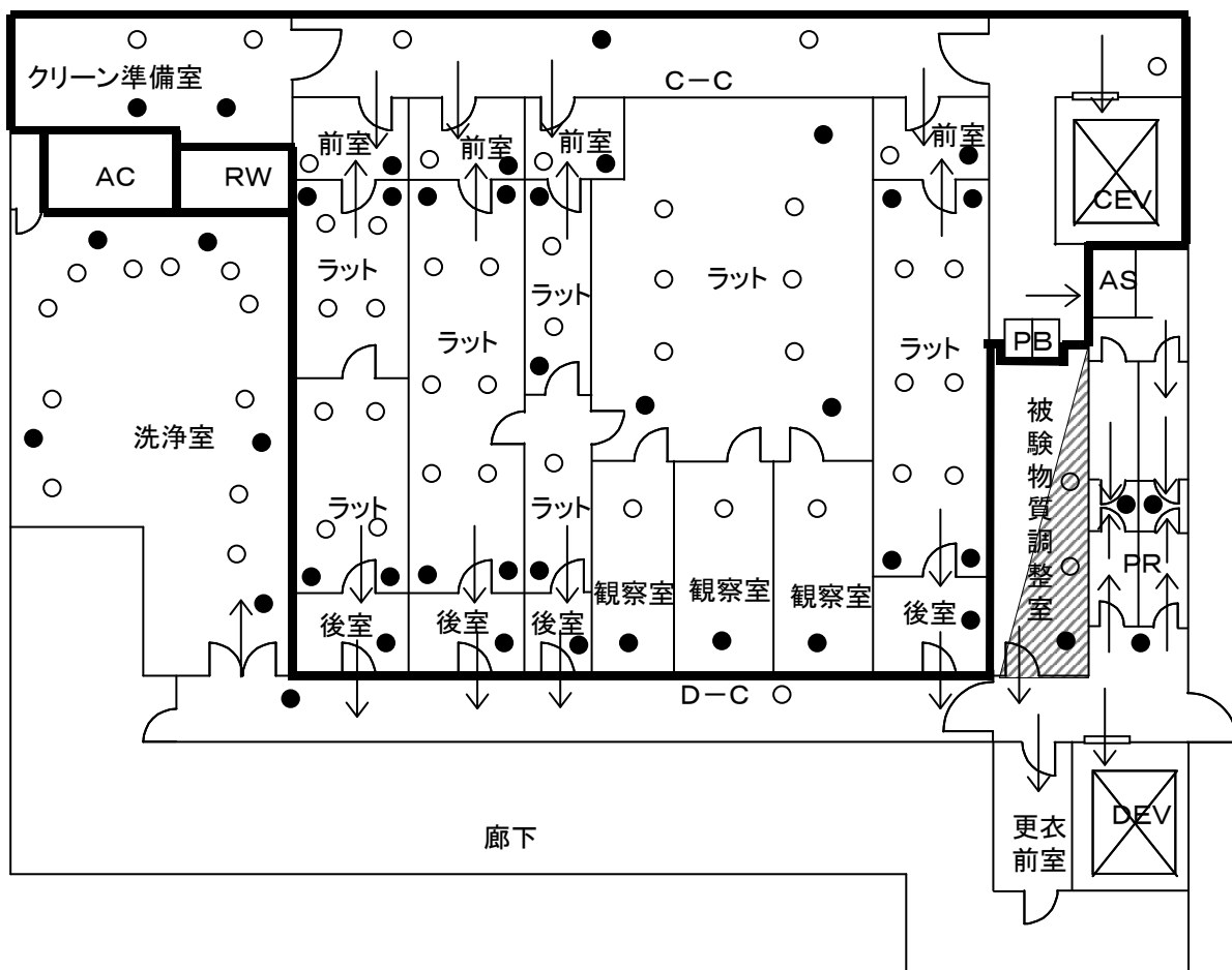
(例) 施設の空調の概略図
