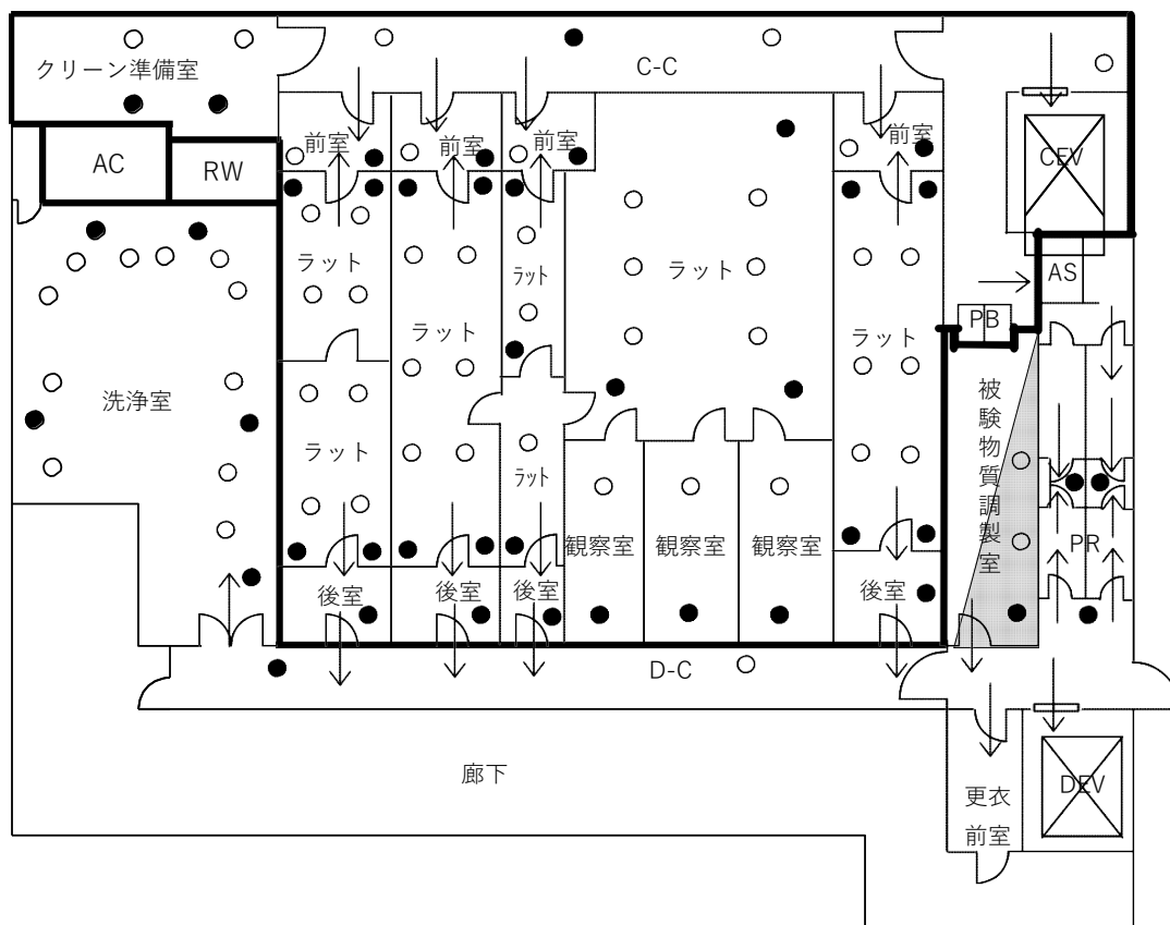
(例) 施設の空調の概略図
