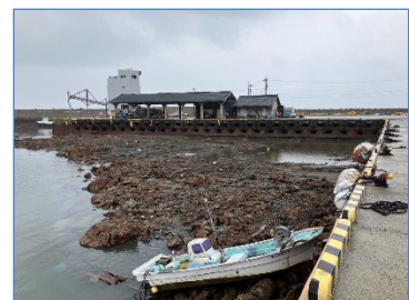
漁港の被害(海底地盤隆起)、漁船の座礁
