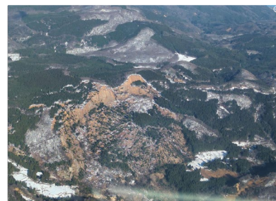
大規模な山腹崩壊
