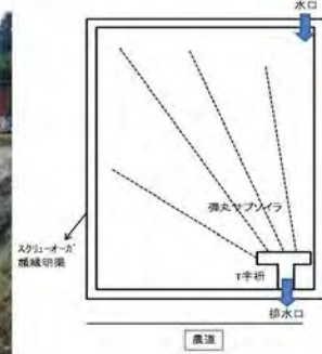
排水対策(集水樹+弾丸暗渠+額縁明渠)の施工
