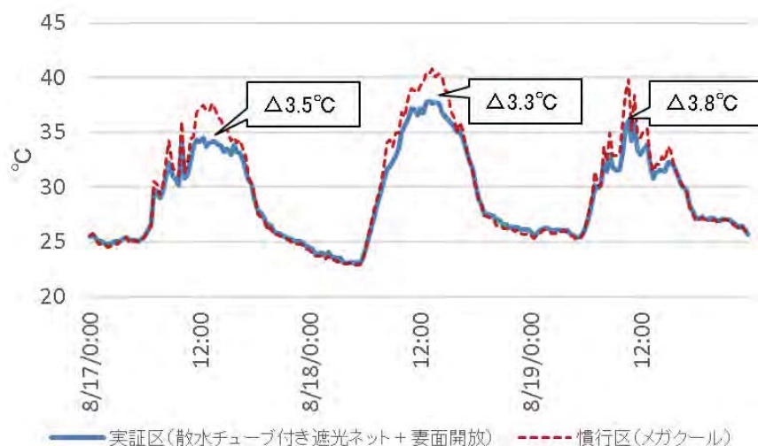
図8 散水チューブ付き遮光ネット+妻面開放ハウスにおける温度の推移 (H30)
