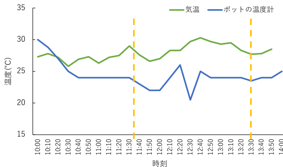
グラフ 1 N.RECSにおける冷却運転時の温度の推移
