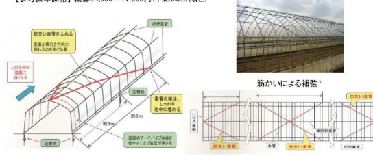
筋かいによる表面の補強方法事例
