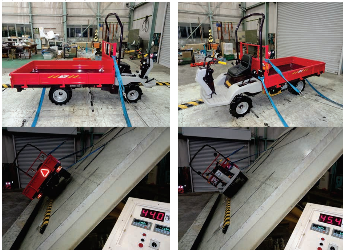
①空車時の左右方向の静的転倒角（左下：左側 2 次転倒、右下：右側 2 次転倒）
