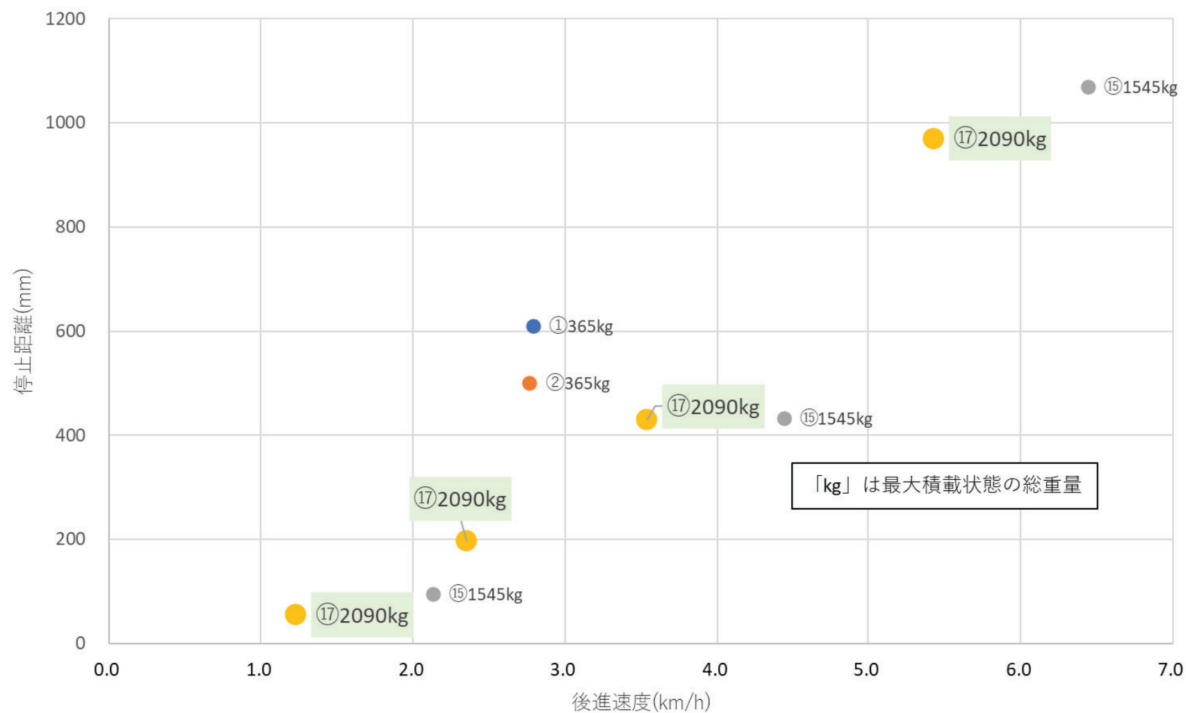
図2 最大積載状態における歩行後進速度および停止距離の比較 ※走行クラッチ操作時
