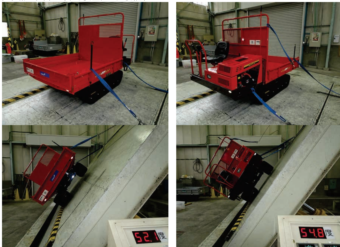
①空車時の左右方向の静的転倒角（左下：左側転倒、右下：右側転倒）
