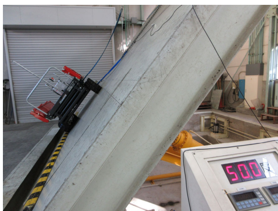
左写真：左方向安定角測定、右写真：右方向安定角測定（安全のため 50° で試験終了）
