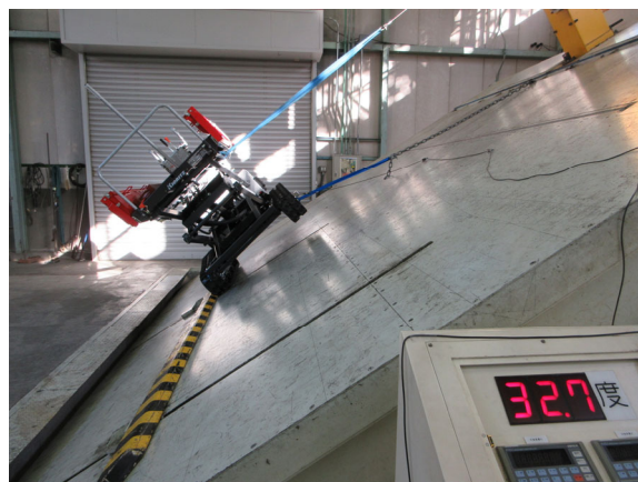
左写真：右方向不利時の左右分担荷重測定、右写真：右方向安定角測定
