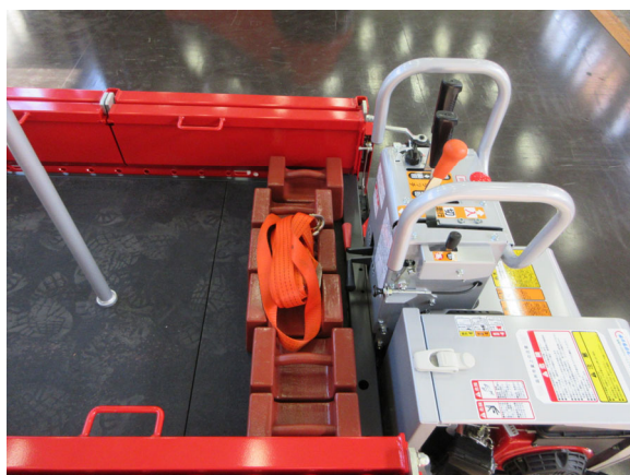
左写真：後方向不利時の左右分担荷重測定、右写真：後方向安定角測定
