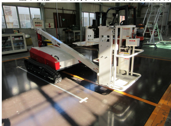
左写真：左右分担荷重測定、右写真：傾斜台への設置状況（チェーン・スリング等で転倒防止）
