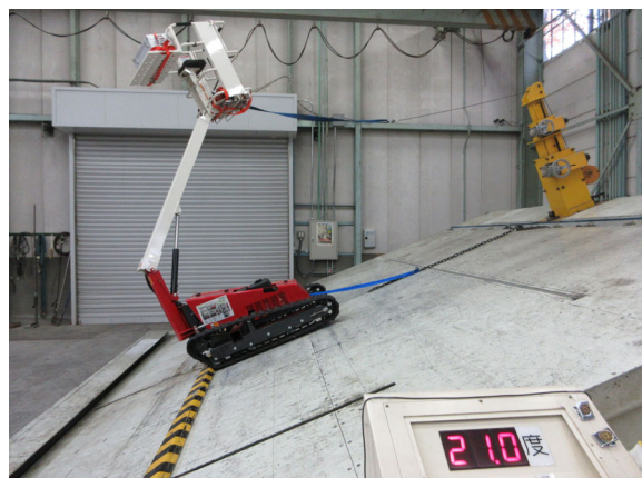
【ブーム角度最大】左写真：前方向不利時の左右分担荷重測定、右写真：前方向安定角測定
