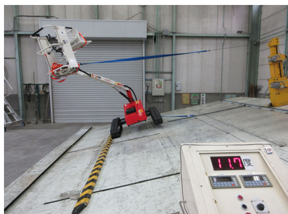
【ブーム角度半分程度】左写真：左方向不利時の左右分担荷重測定、右写真：左方向安定角測定
