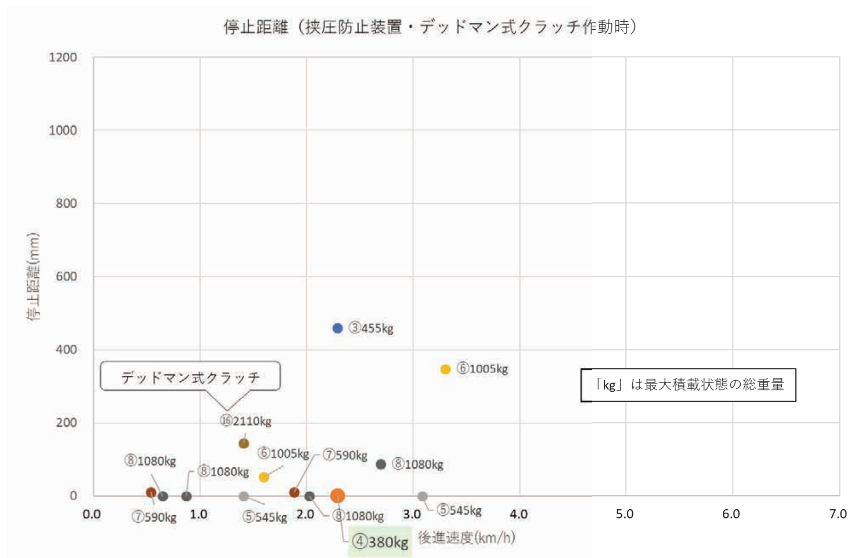
図2 最大積載状態における歩行後進速度および停止距離の比較 ※挟圧防止装置・デッドマン式クラッチ作動時
