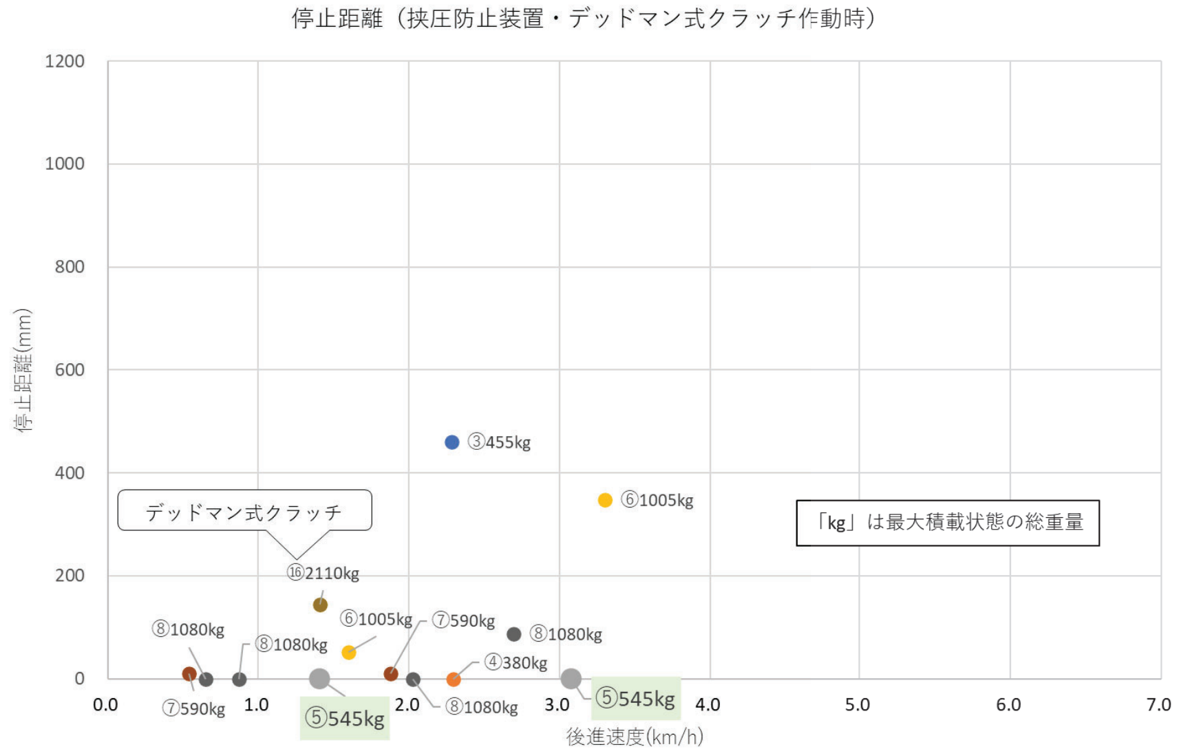
図2-2 最大積載状態における歩行後進速度および停止距離の比較 ※挟圧防止装置・デッドマン式クラッチ作動時
