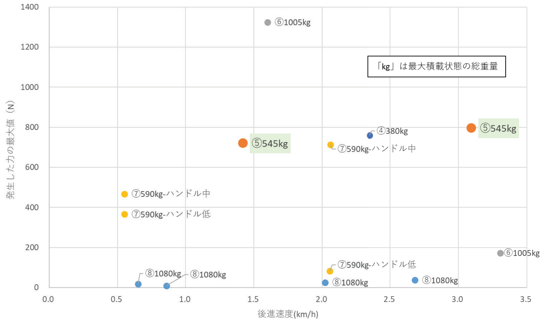
挟圧防止装置作動時に発生した鉛直下向きの力の最大値
