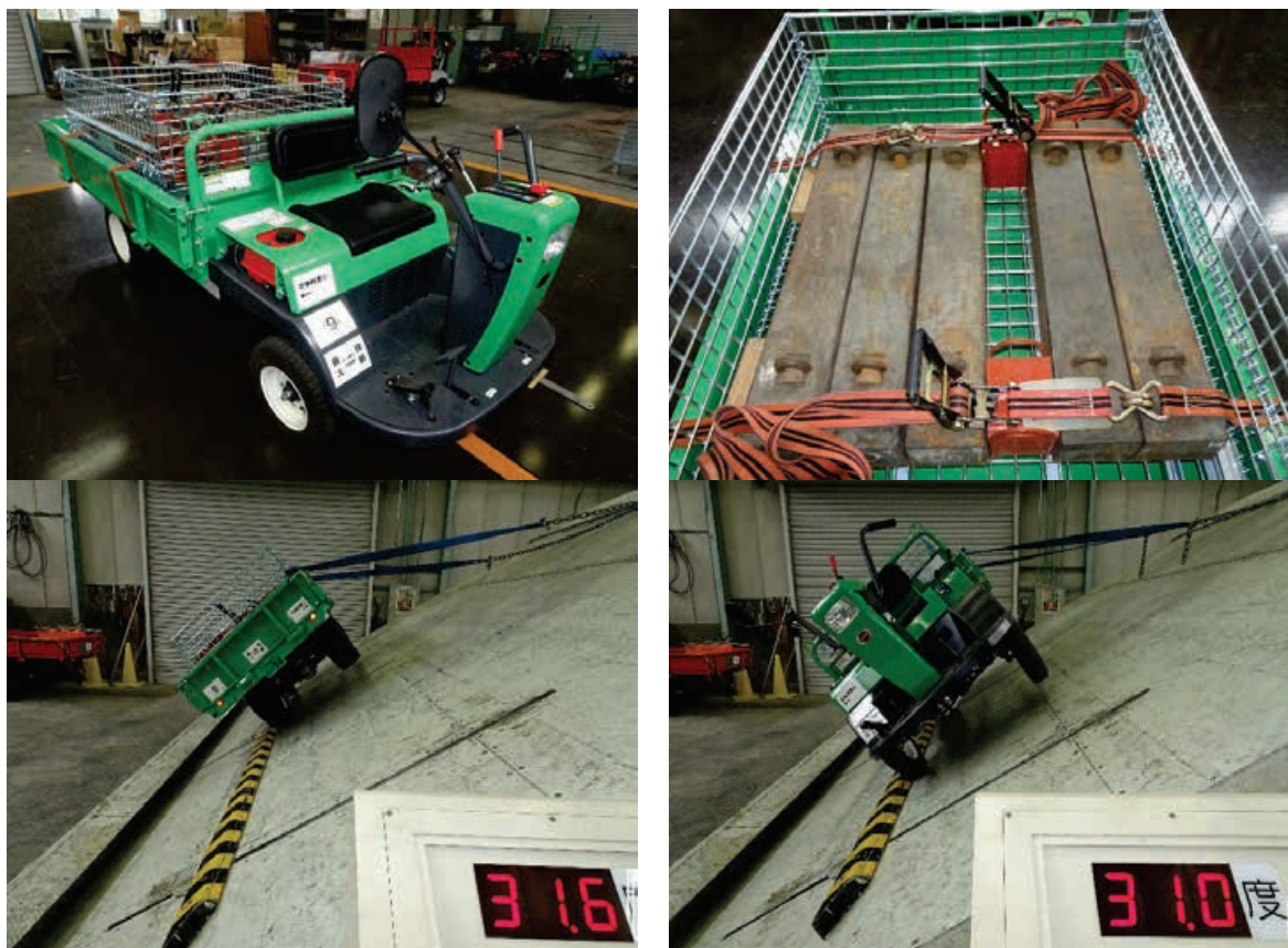
④ばら積みの最大積載状態(等荷重)での左右方向の静的転倒角(左下：左側2次転倒、右下：右側2次転倒)
