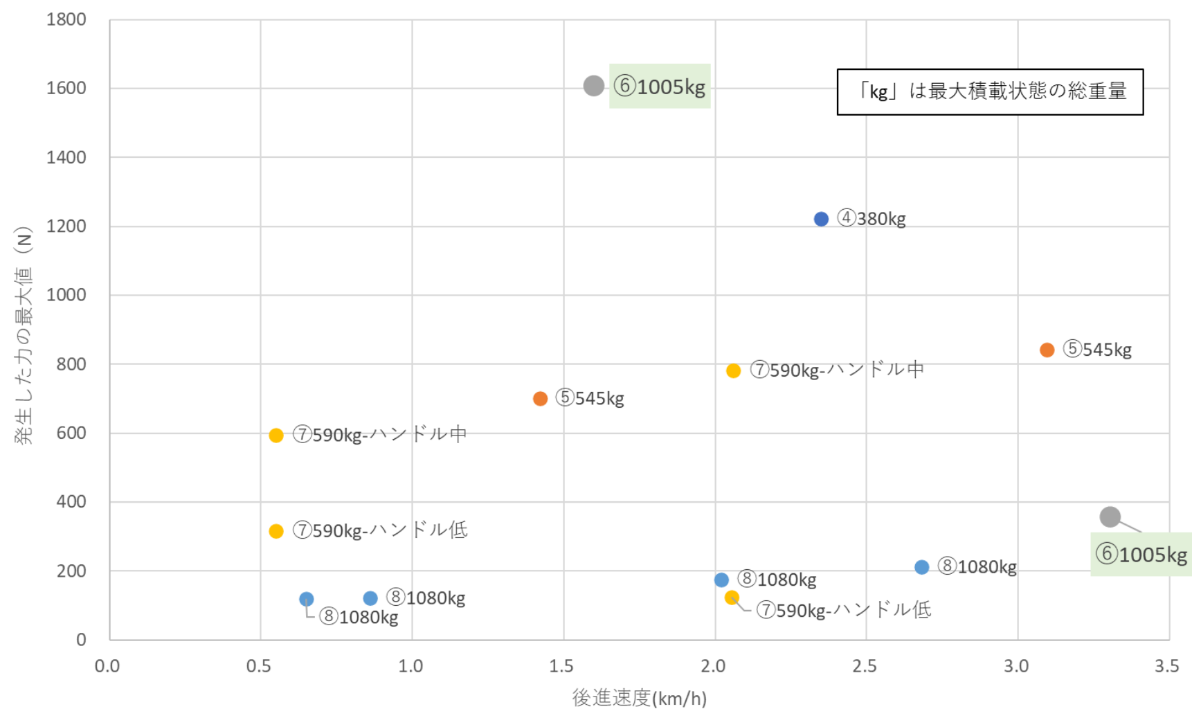
挟圧防止装置作動時に発生した水平方向の押される力の最大値
