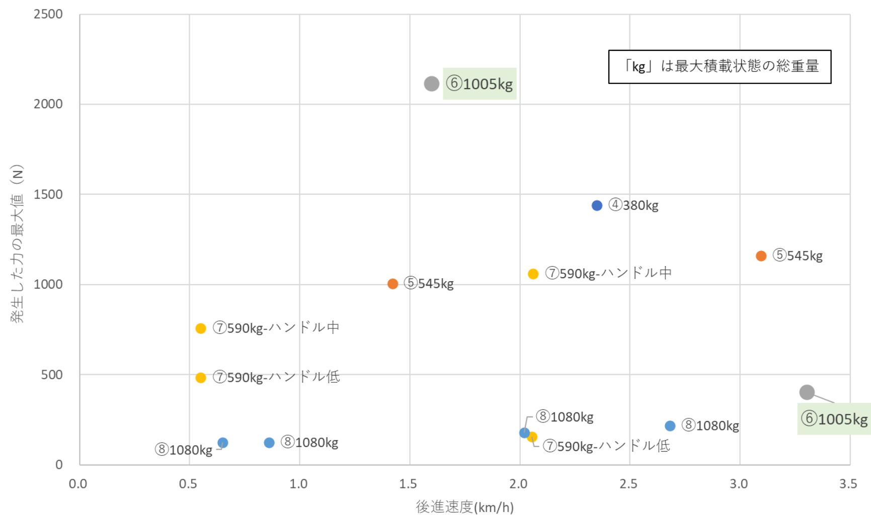
挟圧防止装置作動時に発生した3軸方向の力の合成値（最大値）
