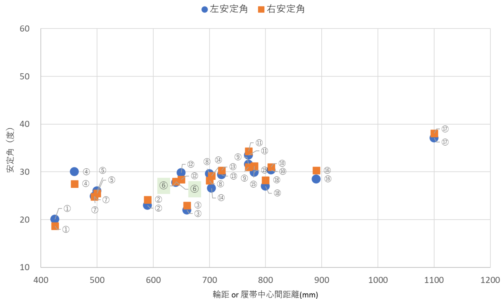
図 1-4 転落・転倒に対する安全性（左右方向の静的転倒角）の比較（18 型式）※ばら積み最大積載等荷重
