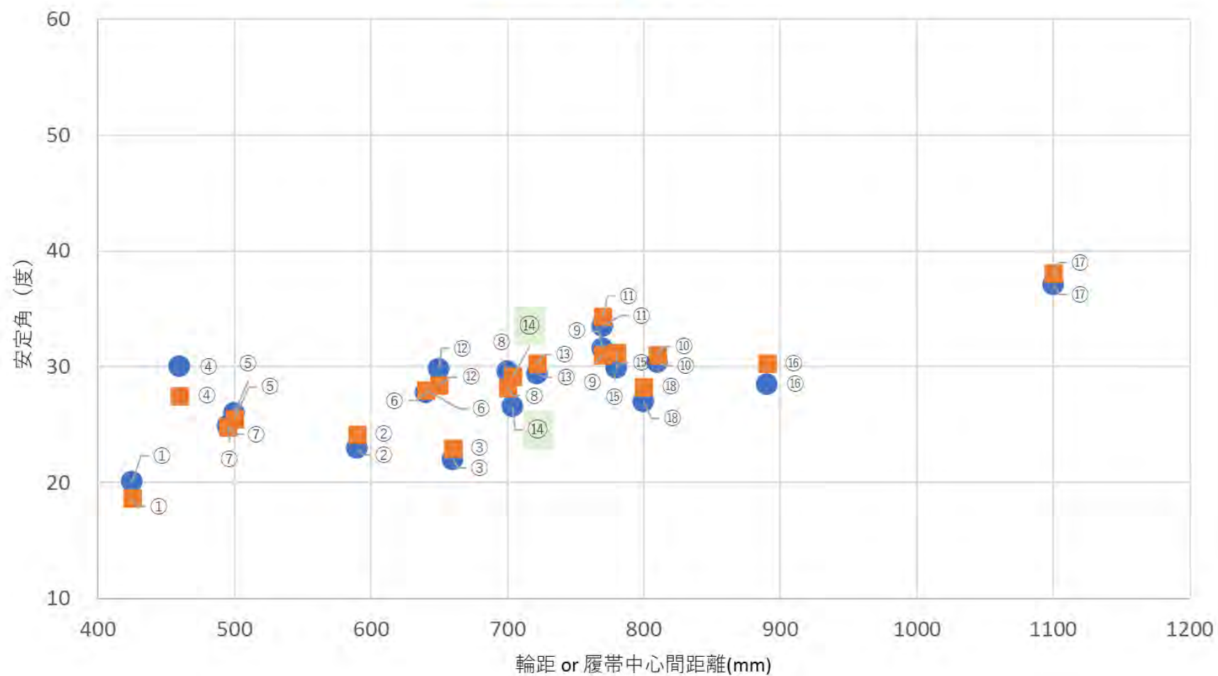
図 1 - 4 転落・転倒に対する安全性（左右方向の静的転倒角）の比較（18 型式）※ばら積み最大積載等荷重
