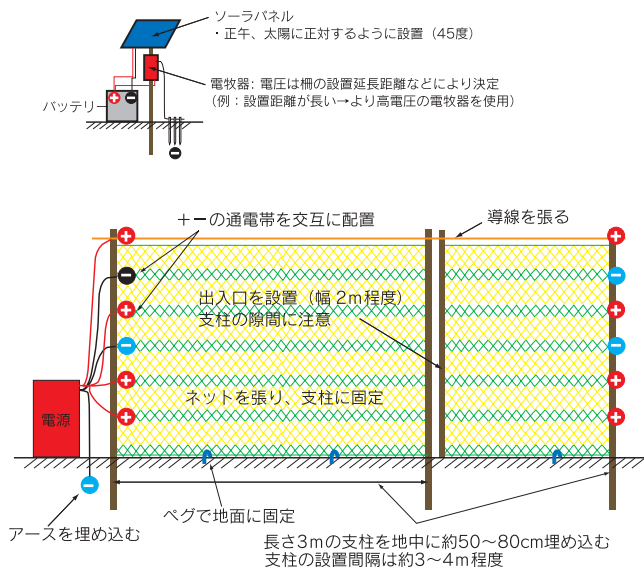
図3.18 従来型のサル用電気ネット柵（正面図）
