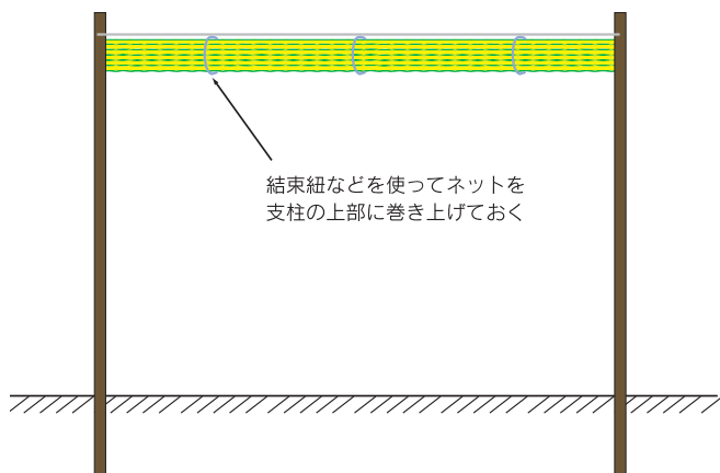
図3.19 冬季のネット型電気柵の管理法
