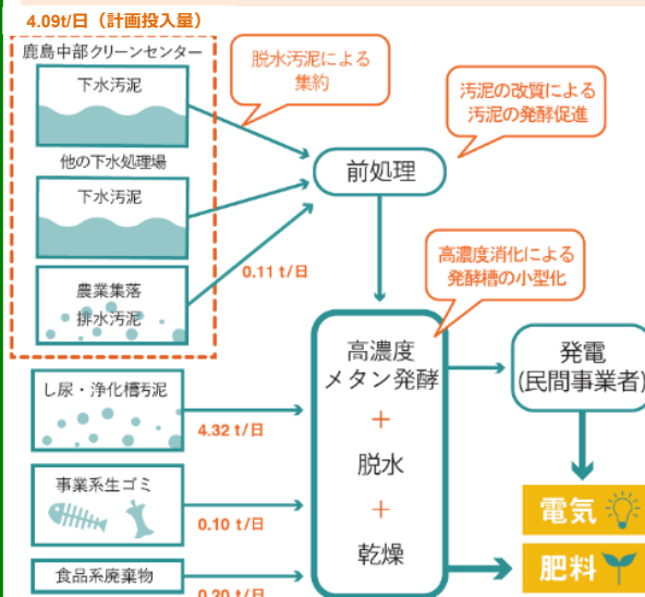
ガス発電設備とメタン発酵槽
