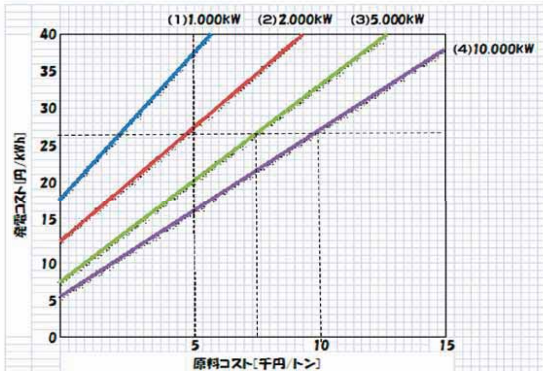
(図5) 発電規模別の事業採算性
