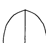
鈍形 (obtuse)
