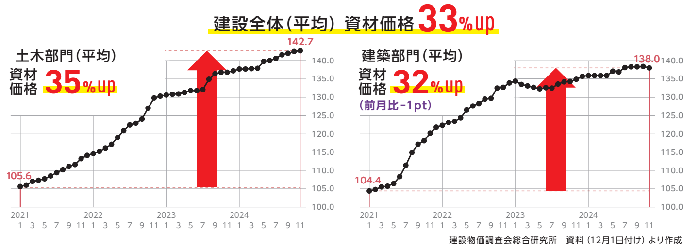
2021年1月～2024年11月の建設資材物価指数(東京)の推移 (2015年平均=100)
