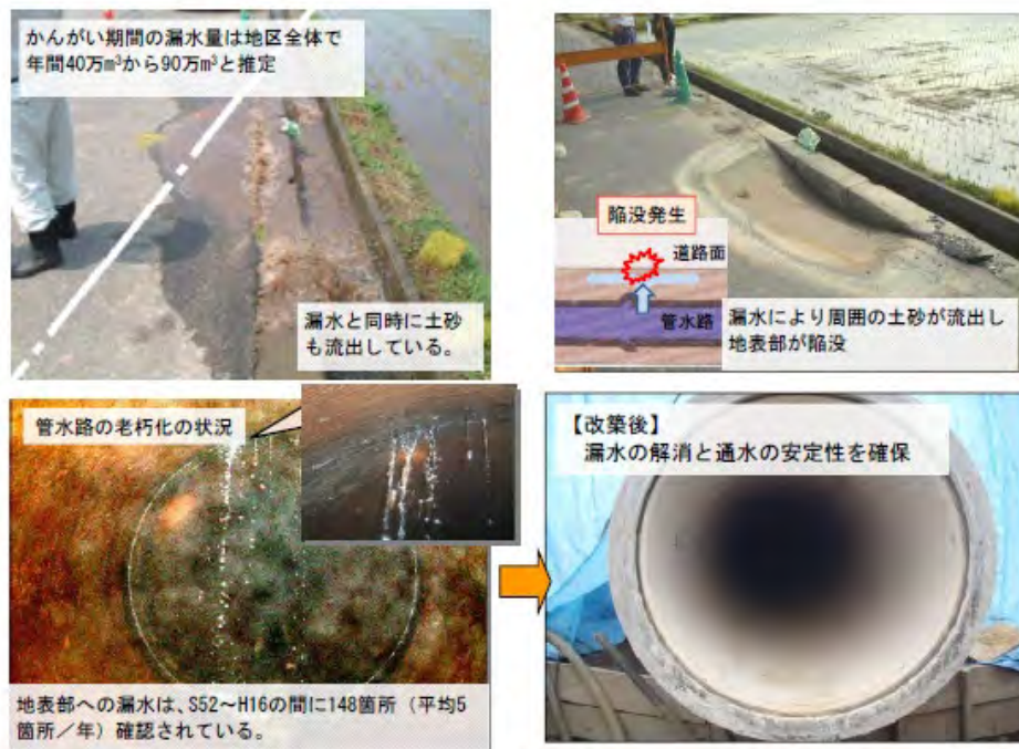
図 幹支線水路老朽化状況及び補修状況
