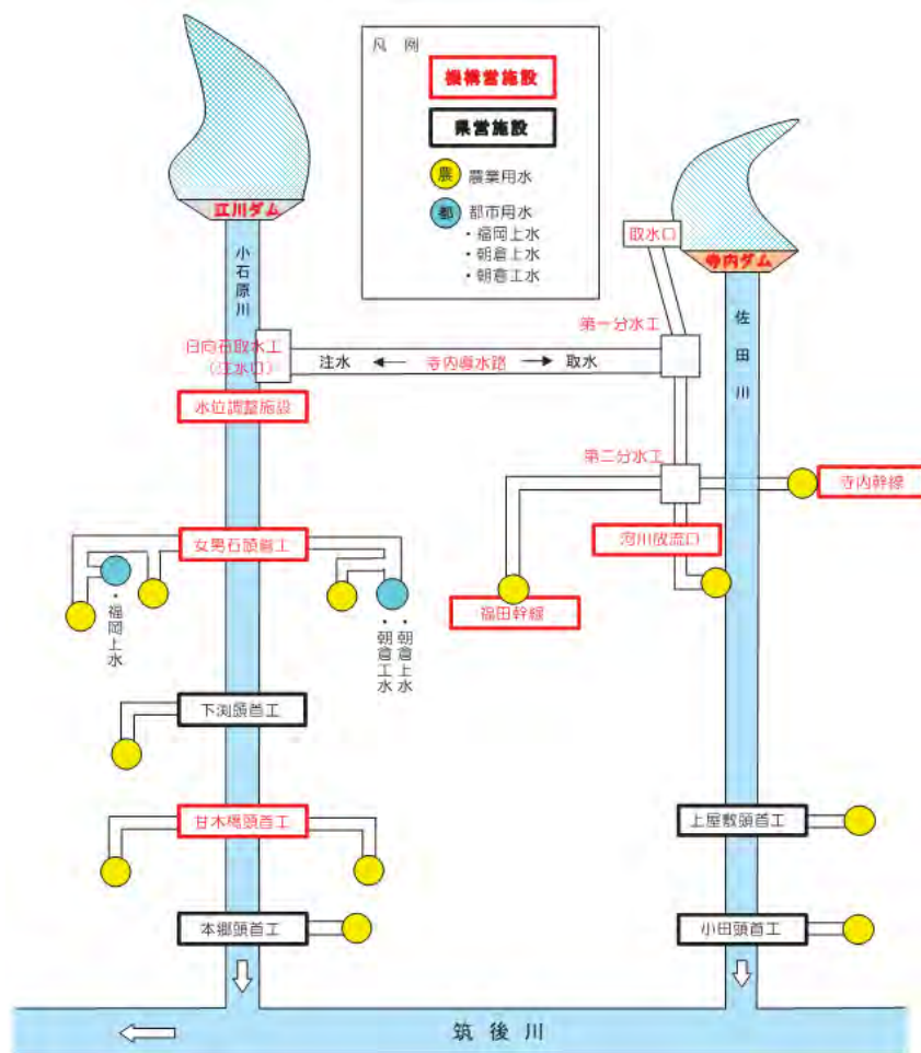
図 小石原川及び佐田川における取水・配水模式図
