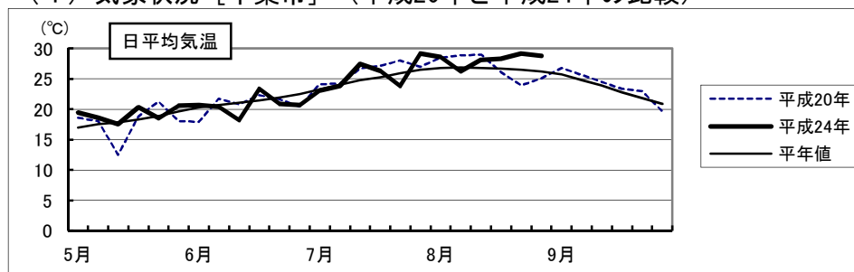
(1) 気象状況〔千葉市〕（平成20年と平成24年の比較）
