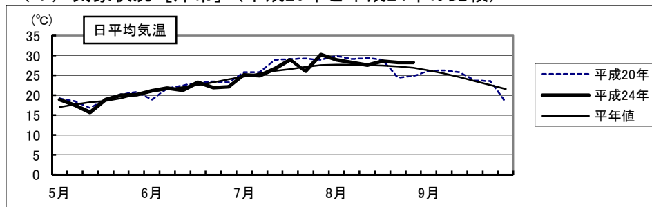
(1) 気象状況〔津市〕(平成20年と平成24年の比較)
