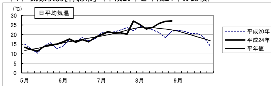
(1) 気象状況[青森市] (平成20年と平成24年の比較)
