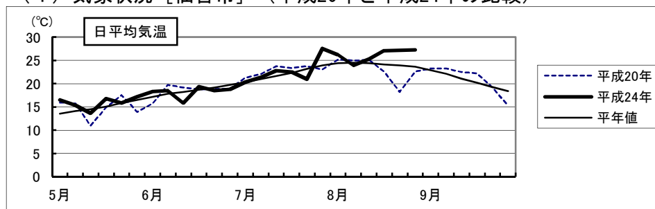
(1) 気象状況〔仙台市〕（平成20年と平成24年の比較）
