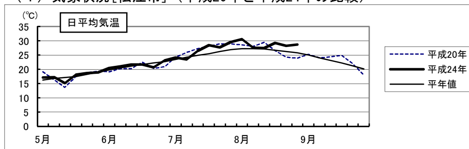
(1) 気象状況[松江市] (平成20年と平成24年の比較)
