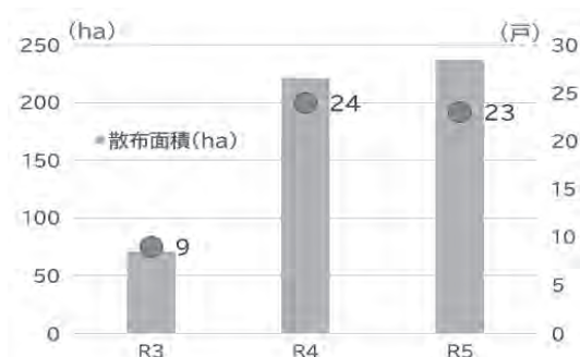
図2 消化液の利用戸数と散布面積の推移 (上士幌町耕種農家)
