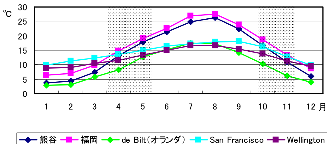
図1 Phytophthora ramorum 及び P. kernoviae の分布地域と日本（熊谷、福岡）の月別平均気温の比較
