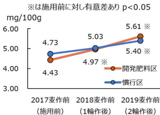
土壌中可給態窒素量の推移
