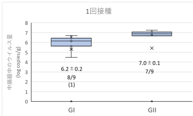
図7. 海水へのノロウイルス接種を1回にした場合のカキ中腸腺中のノロウイルス量
