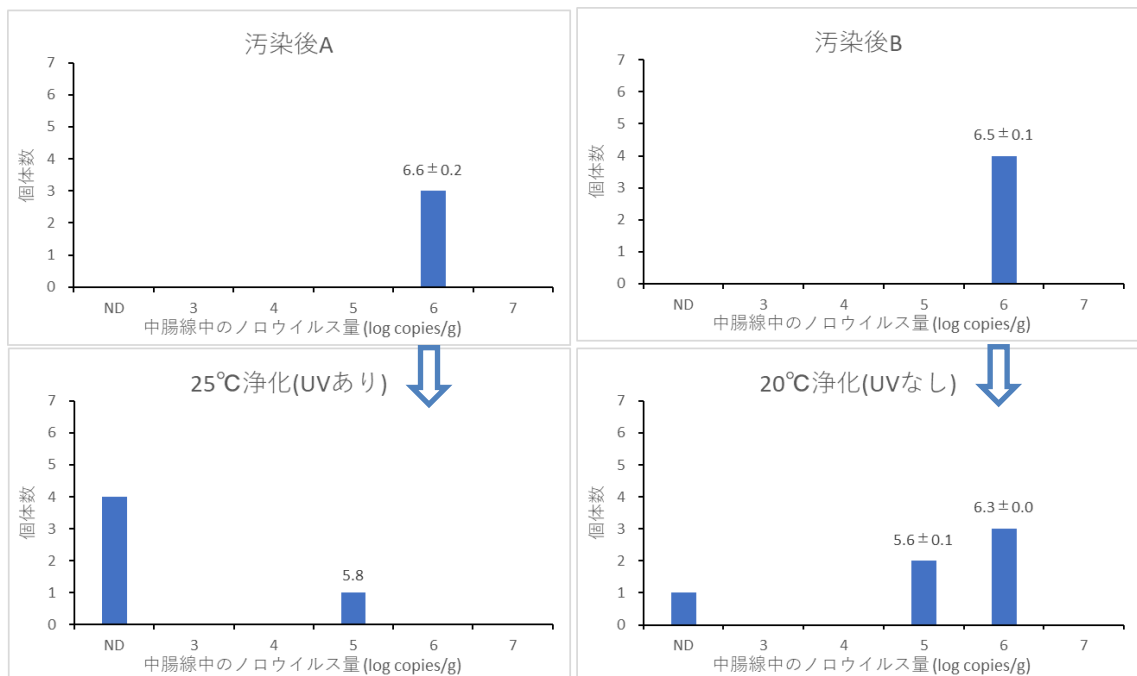
図21. 高濃度汚染後(上段)および20℃・25℃海水で浄化後(下段)のカキ中腸腺中のノロウイルスGII量
