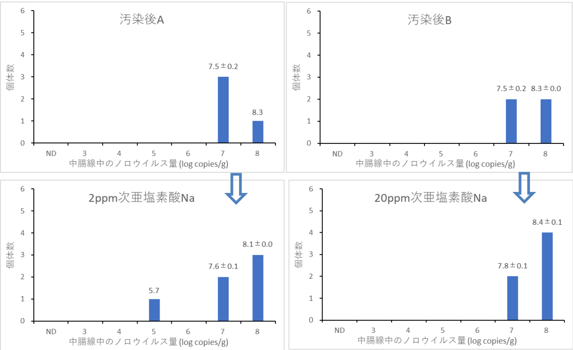
図23. 高濃度汚染後(上段)および次亜塩素酸Na添加海水で浄化後(下段)のカキ中腸腺中のノロウイルスGI量
