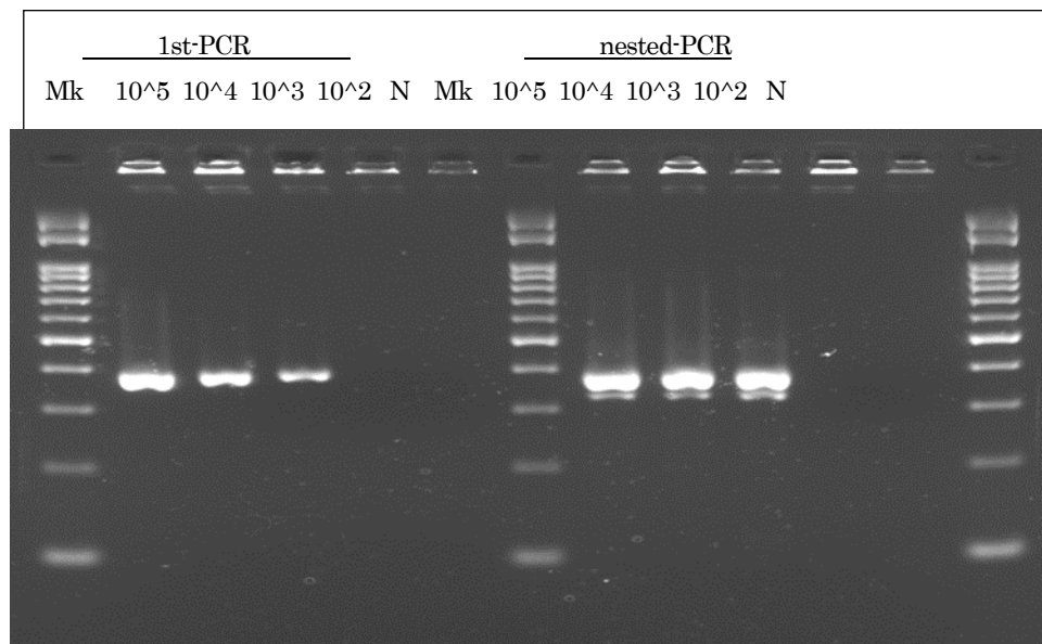
図17. PEG6000およびCMC-Naを共沈材として用いた海水からのノロウイルス回収方法の検出感度
