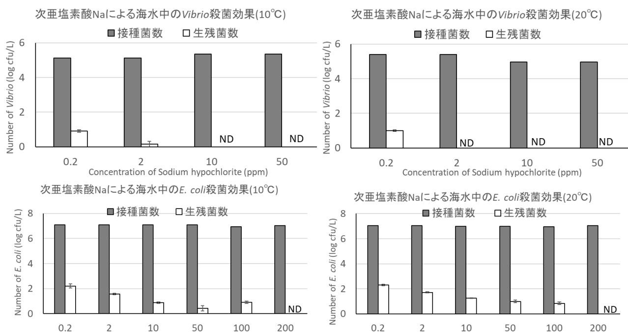
図16. 次亜塩素酸ナトリウム処理による海水中の腸炎ビブリオおよび大腸菌への殺菌効果
