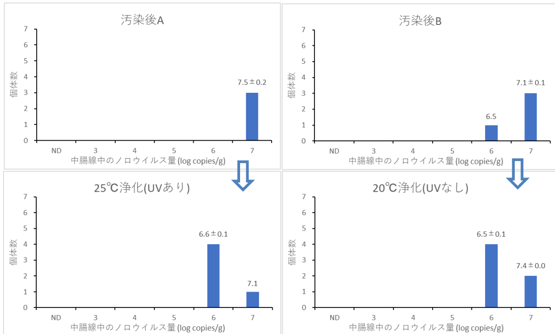
図20. 高濃度汚染後(上段)および20℃・25℃海水で浄化後(下段)のカキ中腸腺中のノロウイルスGI量
