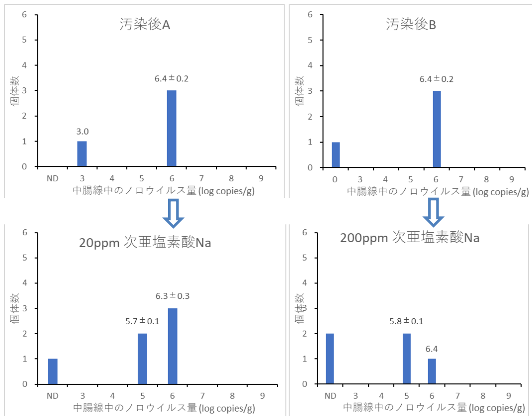
図26. 高濃度汚染後(上段)および次亜塩素酸Na添加海水で浄化後(下段)のカキ中腸腺中のノロウイルスGII量(2回目)
