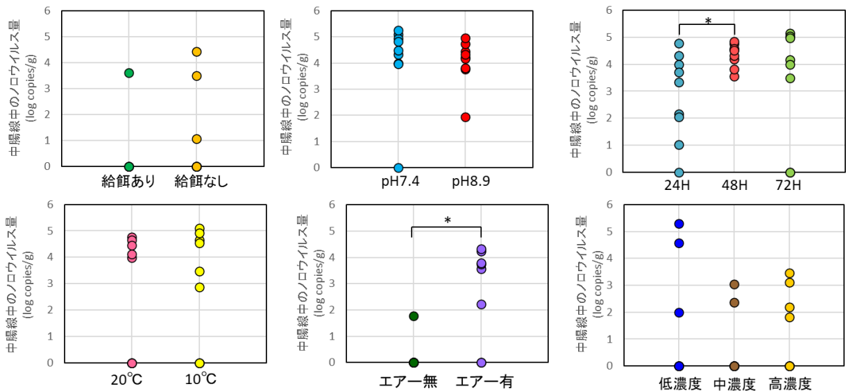
図1. 各種飼育環境下におけるノロウイルス蓄積量(GII. 4)
