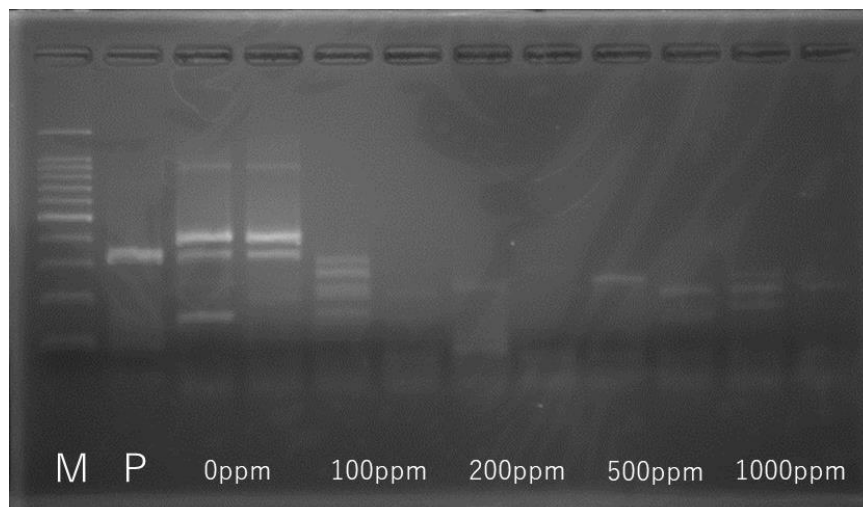
図18. 海水中のノロウイルス不活化試験の電気泳動結果
