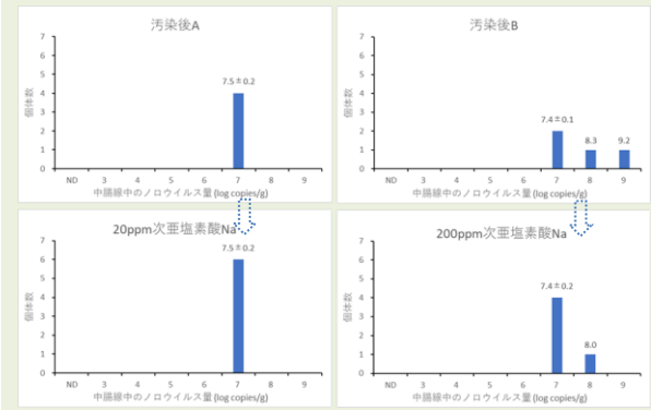
図 2. 20ppmおよび200ppmの次亜塩素酸ナトリウムを添加した海水中でカキを浄化した際の中腸腺中のノロウイルス量 (ノロウイルスGI.7) (上段)浄化前カキ試料のノロウイルス量 (下段)浄化後のカキ試料のノロウイルス量 200ppmの次亜塩素酸ナトリウムを含む海水中で畜養しても中腸腺中のノロウイルスは低減しなかった。
