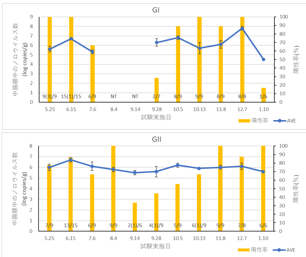
図11. 月別カキのノロウイルス蓄積量および陽性率の変化(2022-2023シーズン)
