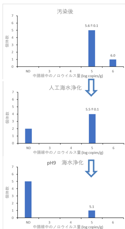
図22. 高濃度汚染後(上段)およびpH9.05・通常の人口海水で浄化後(下段)のカキ中腸腺中のノロウイルスGII量
