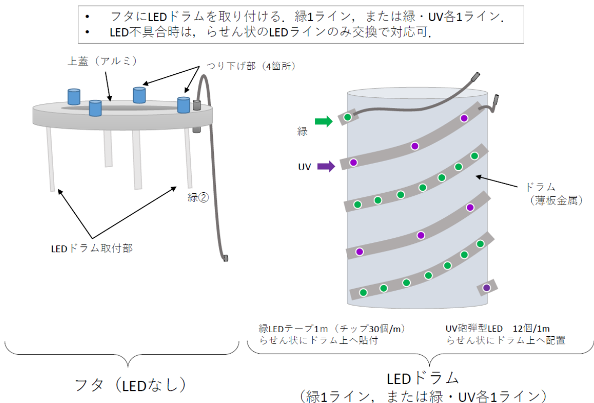
図7 光源セットを構成する、フタ（左）とLEDドラム（右）
