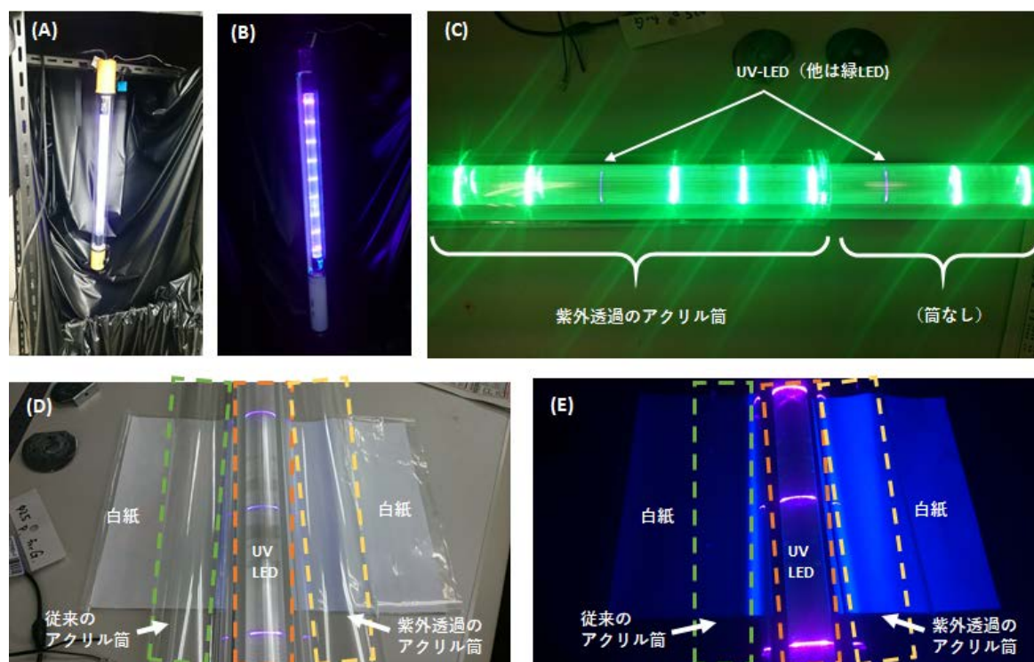
図 8 20 W 蛍光灯器具とそれに取り付けられた LED 光源 (A) (B)、及び、その外筒であるアクリル筒の紫外透過検討。(C) 紫外透過のアクリル筒を UV-LED を含む蛍光灯形 LED を半分カバーし、アクリル筒があるところでも UV-LED の光が透過していることがわかる。(D) 中央に蛍光灯形 UV-LED を置き、その左側に紫外線吸収剤添加の従来アクリル筒、右側に紫外線透過アクリルを置き、照明を消すと、(E) 紫外透過アクリル側のみ、下に敷いてある白い紙が紫外線による蛍光を発しており、紫外線が透過していることがわかる。
