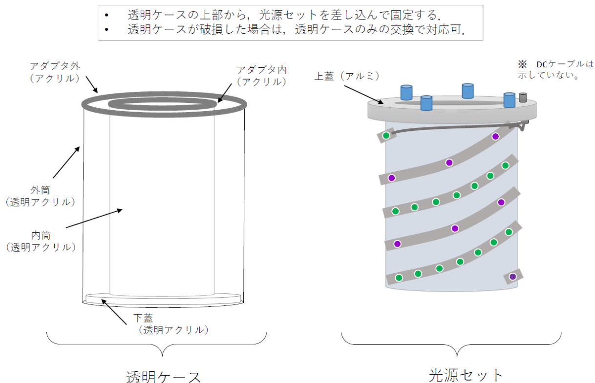
図6 LED 光源装置を構成する、透明ケース（左）と光源セット（右）
