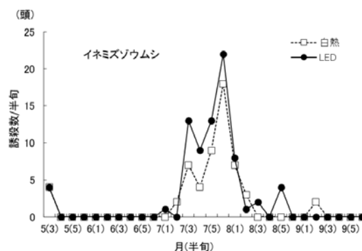
図5 イネミズゾウムシの誘殺消長
