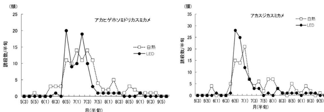
図6 斑点米カメムシ類の誘殺消長
