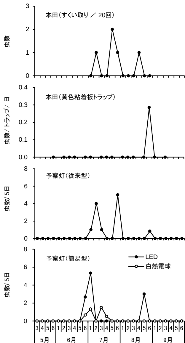
図2 ヒメビウカの発生消長と予察灯の誘殺消長
