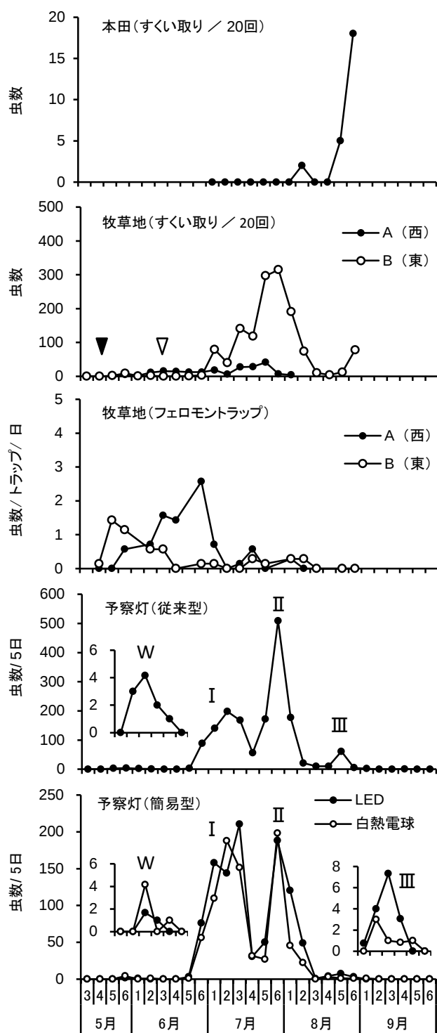
図7 アカヒゲホソミドリカスミカメの発生消長と予察灯の誘殺消長
