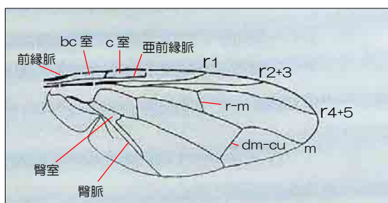
図7 ミバエの翅
