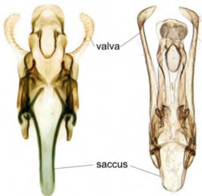
図 13 トマトキバガ(左)とジャガイモガ(右)の雄交尾器 (防疫指針委託事業成果)
