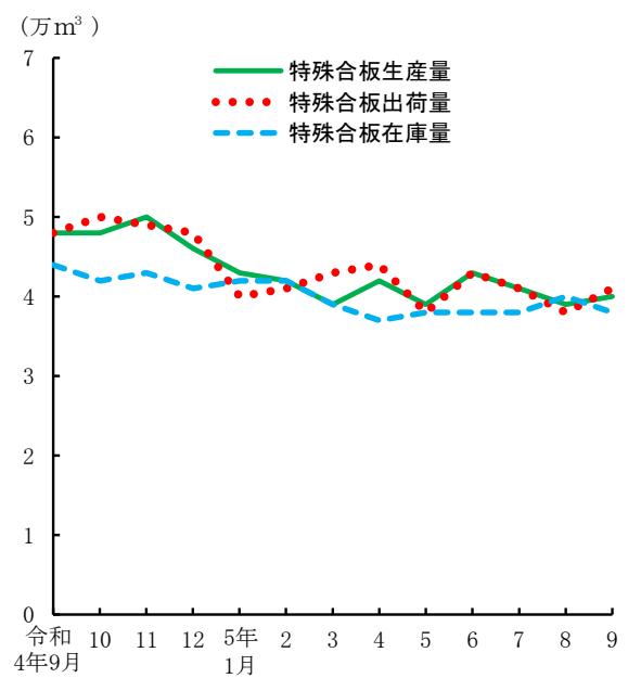
図2 特殊合板の生産量、出荷量及び在庫量の推移
