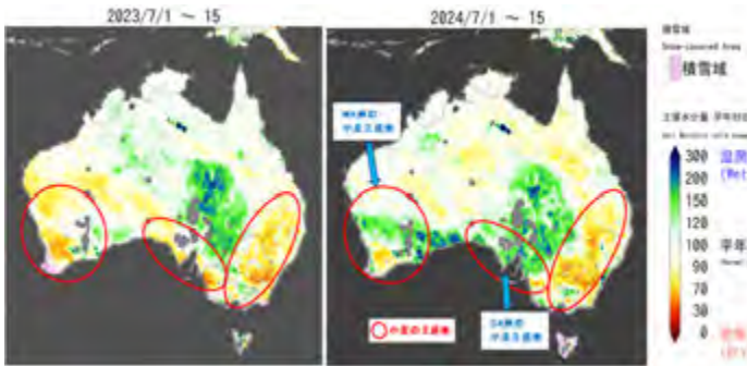
図 豪州の土壌水分量 「前年に比べ WA 州、SA 州で土壌水分が改善」
