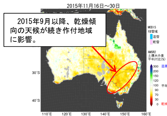
【図2】北米の乾燥状況(図1の参考) 【図3】豪州の乾燥状況(図1の参考)
