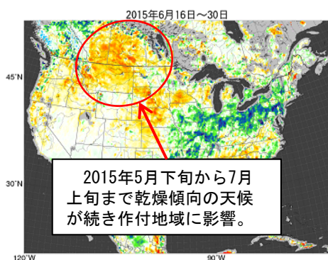
【図2】北米の乾燥状況(図1の参考) 【図3】豪州の乾燥状況(図1の参考)
