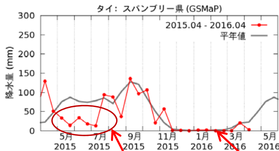
【図2】タイの降水量・乾燥状況(図1の参考)
