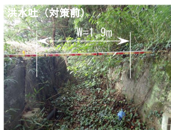
流下能力が不足した洪水吐・放水路
