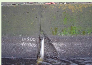
水路目地部の破損
