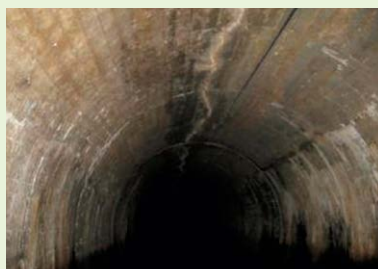
導水幹線暗渠部のクラック
