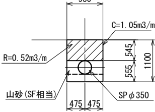
C-C断面 S=1 : 50
