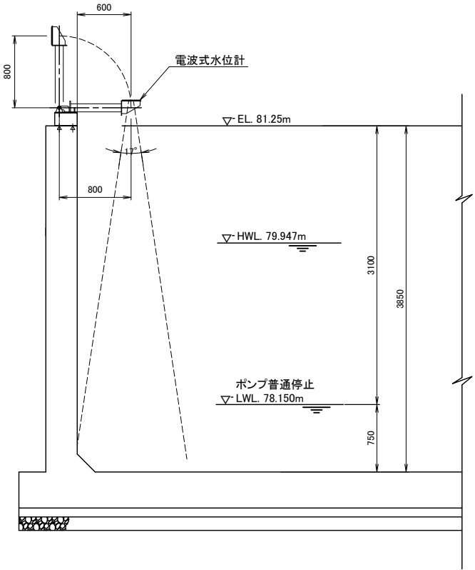
断面図 S=1:30
