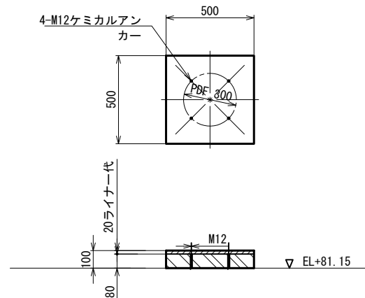
圧カタンク基礎詳細図 S=1:15
