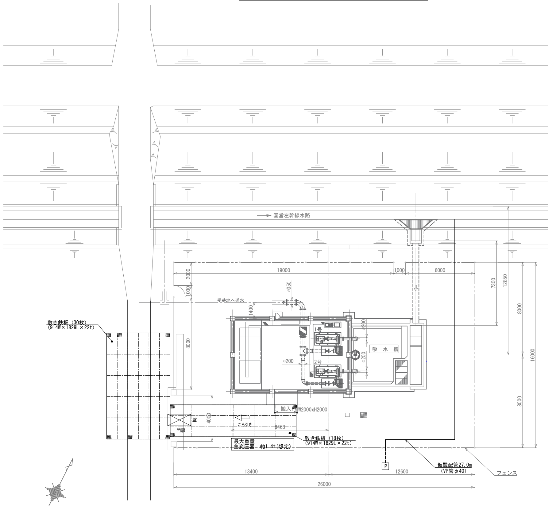
櫛挽第 1 揚水機場 仮設計画図 S=1 : 100
