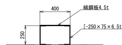
鋼製ケーブルダクト
