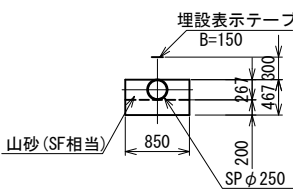
管体工標準断面図 S=1 : 50
