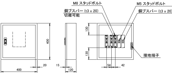
接地端子箱 外形図 S=1:10
