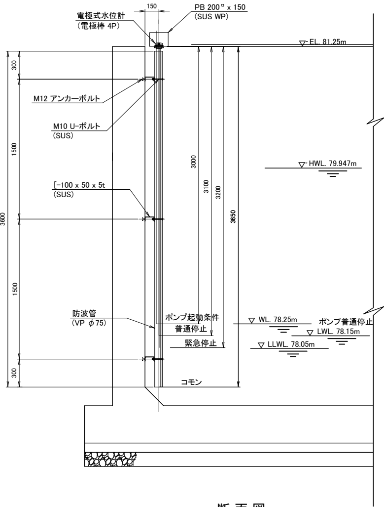
断面図 S=1:20
