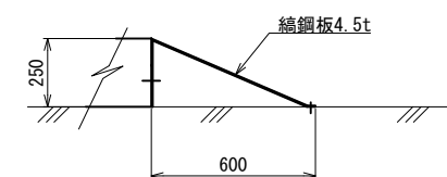
スロープ o S=1:15
