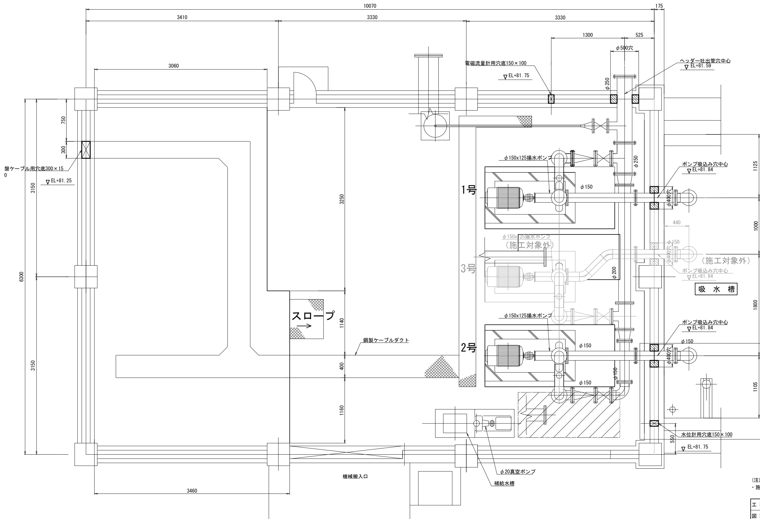
櫛挽第1揚水機場 穴開け図 S=1:20
