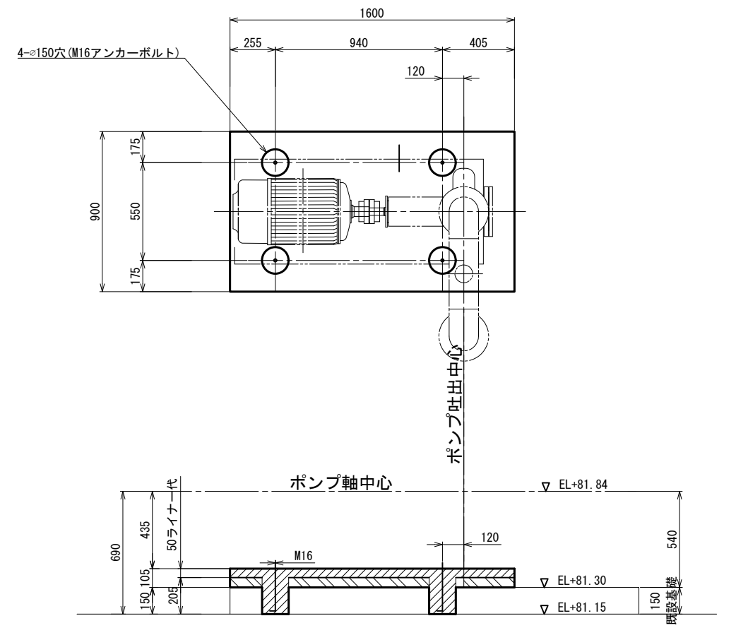
1号・2号揚水ポンプ基礎詳細図 S=1:15
