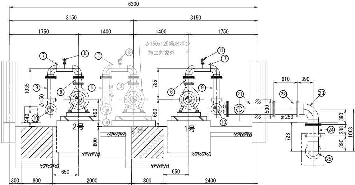
断面 B B
