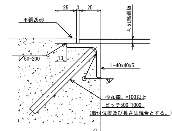
ピットフチ金具 詳細図 S=1:2
