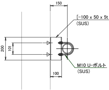
防波管 取付詳細図 S=1:10
