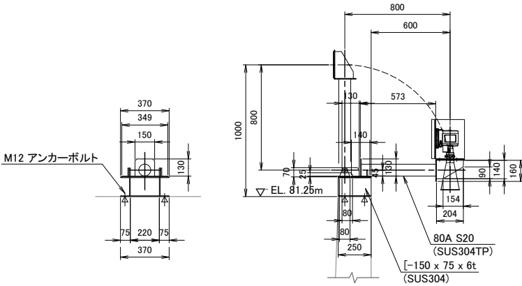
詳細図 S=1:20
