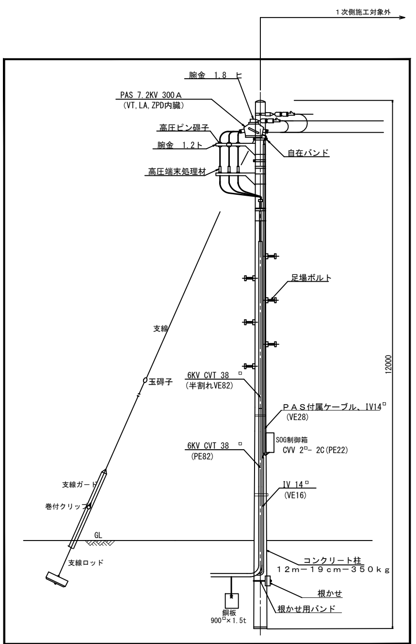
引込装柱図
